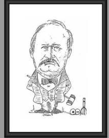
Svante Arrhenius (1859-1927) determinó que la temperatura superficial media de la tierra es de 15^\circ\text{C} debido a la capacidad de absorción de la radiación infrarroja por parte del vapor de agua y del \text{CO}_2 ("efecto invernadero natural"). Arrhenius sugirió que una concentración doble de estos gases de invernadero provocaría un aumento de temperatura de 5^\circ\text{C}
