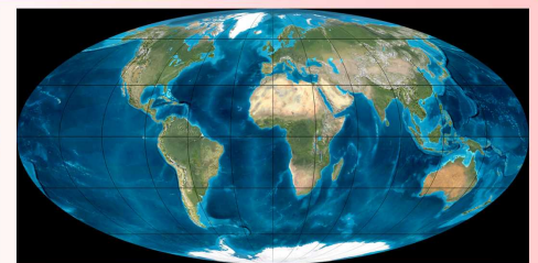
Extensión de hielo en la actualidad
