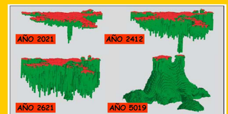
Comportamiento esperado del CO 2 inyectado en una formación geológica. El CO 2 libre (rojo) se va disolviendo (verde) y se hunde en la formación
