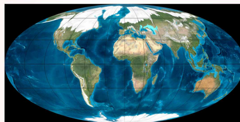
Extensión de hielo en la etapa glacial
